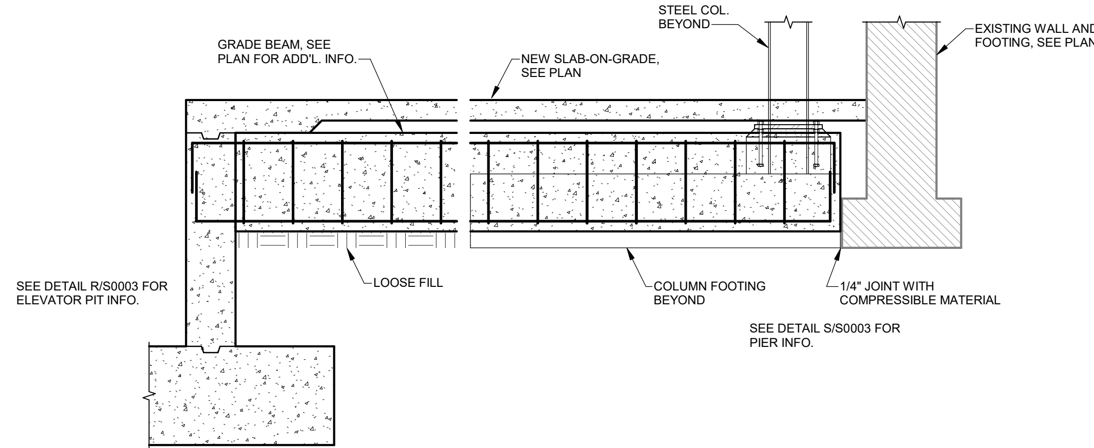
SECTION 8 SCALE: 1/2" = 1'-0"
