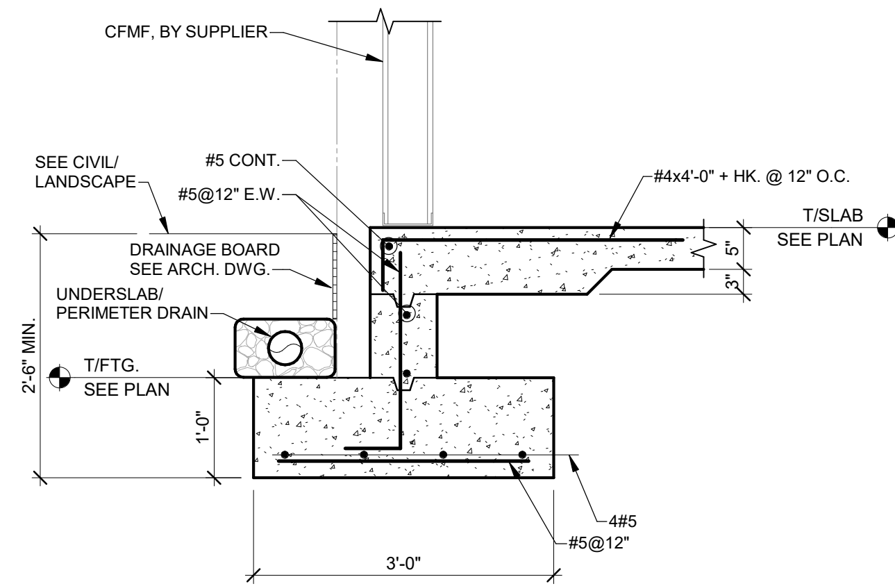
SECTION 7 SCALE: 3/4" = 1'-0"
