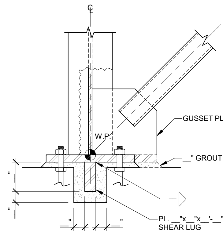
SECTION SCALE: 3/4" = 1'-0"
