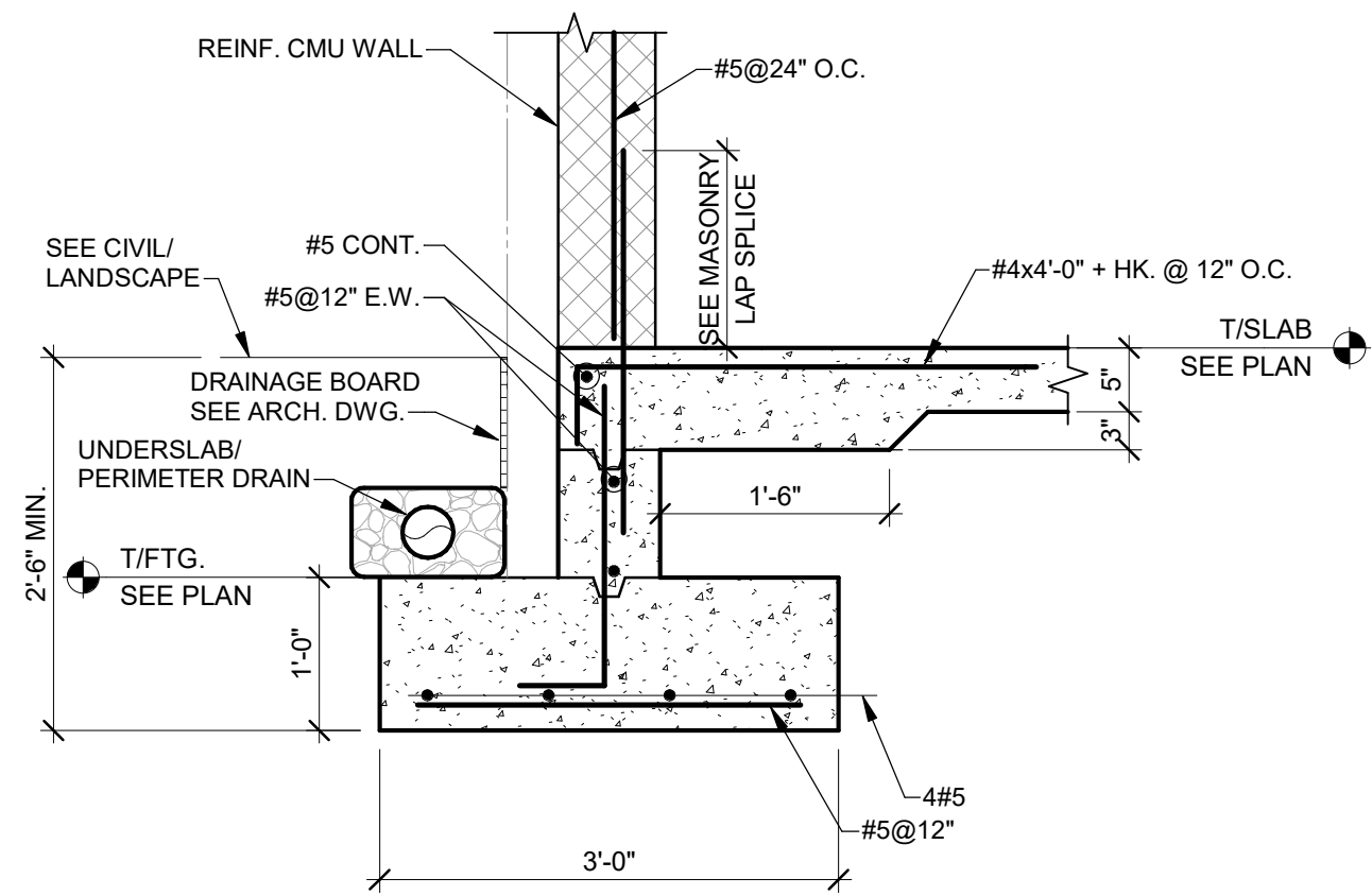
SECTION 6 SCALE: 3/4" = 1'-0"
