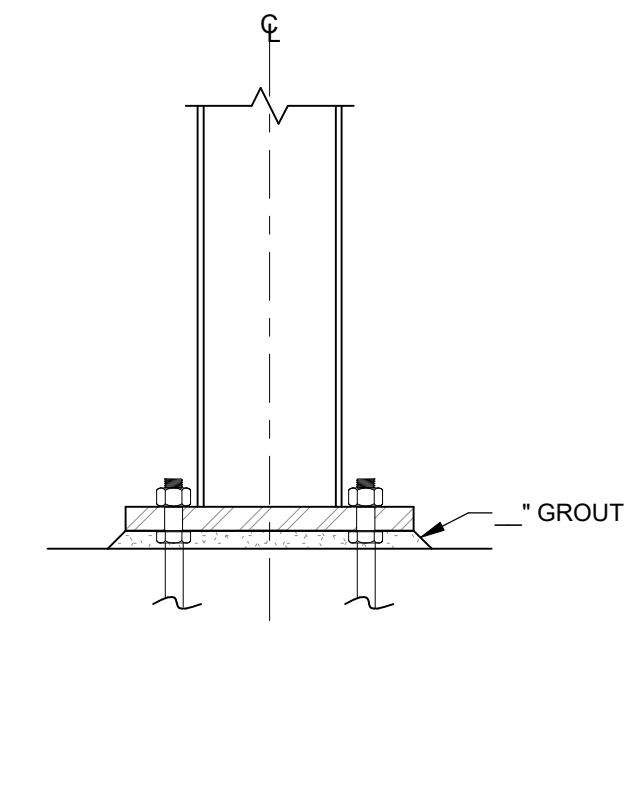
SECTION SCALE: 3/4" = 1'-0"
